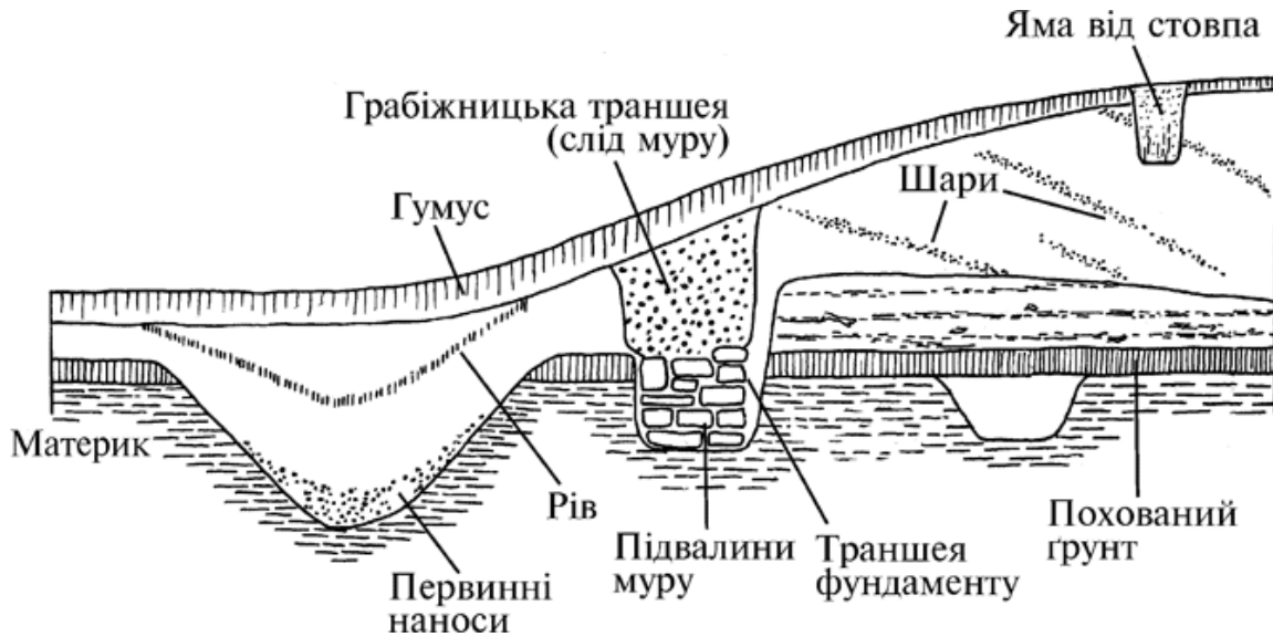
Стратиграфічний розріз
